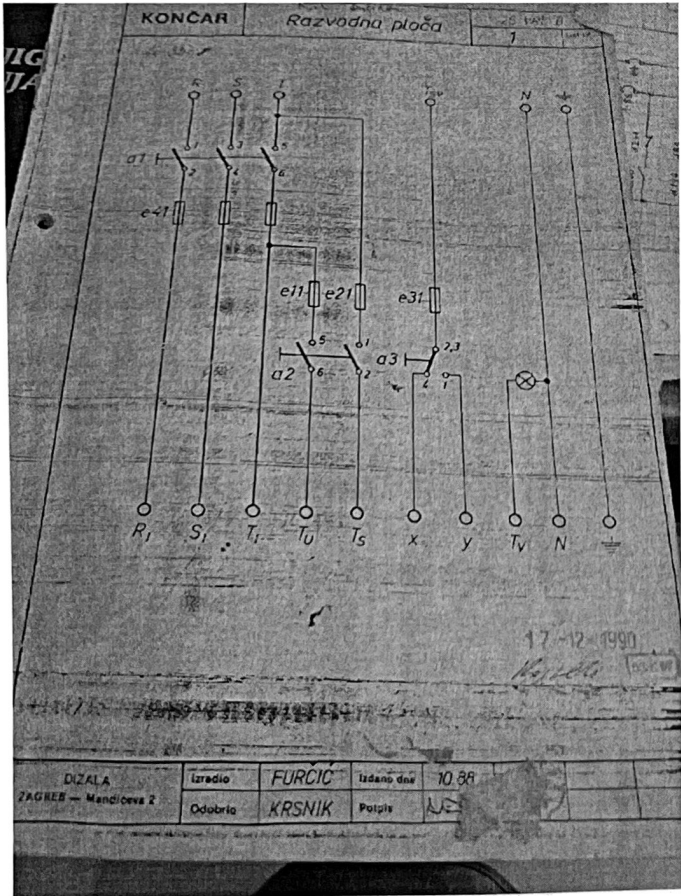
Slika 5. Skica razvodne ploče
